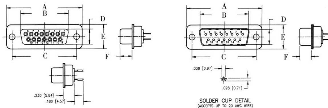
针式/孔式/焊杯式 D 型连接器尺寸表:
