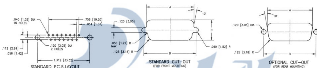
PCB 板安装孔尺寸表:
