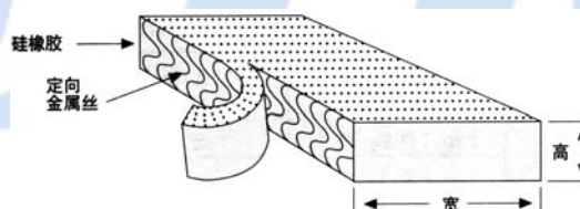
定向金属丝橡胶衬垫结构图
